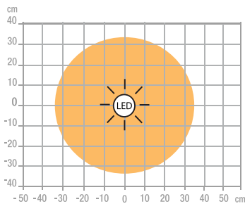
Mesure en Lux sur le plan de travail en vue de dessus à 40 cm:
