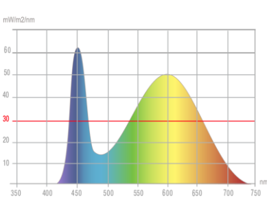
Mesure en nanomètre du spectre lumineux
