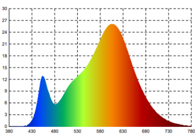
Mesure en nanomètre du spectre lumineux
