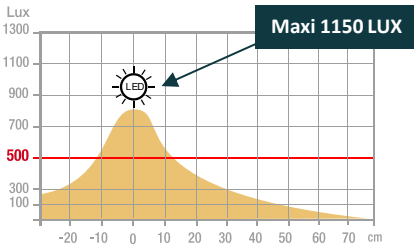
Mesure en Lux sur le plan de travail en vue de profil à 40 cm:
