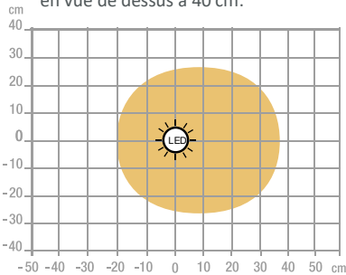
Mesure en Lux sur le plan de travail en vue de dessus à 40 cm:
